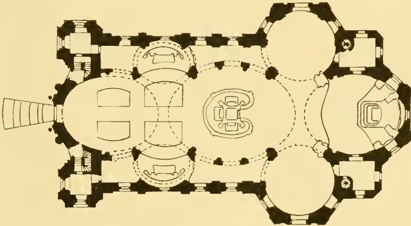
Fig. 113. Kirche zu Vierzehnheiligen. Grundriss.
